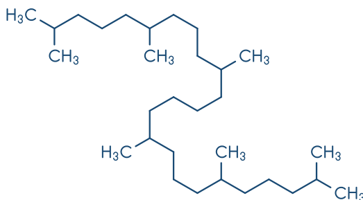
Chemische Struktur von Squalan
